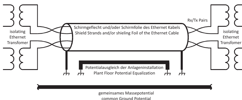
Fig. 15: Equipotential bonding and grounding
